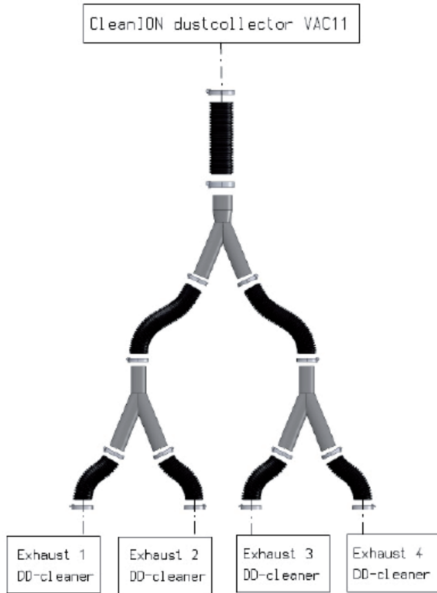
Beispiel Schlauchsets DD-04
