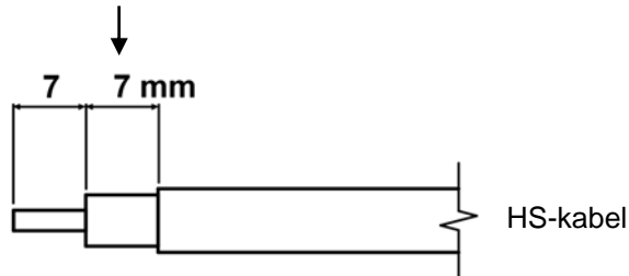
Afbeelding 4: afwerking HS-kabel
