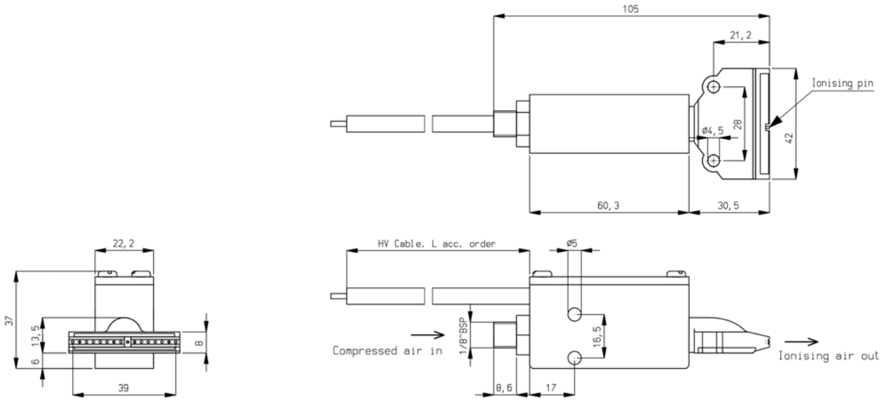
Figure 1 : dépoussiéreur à air ionisé de type FLAT 2
