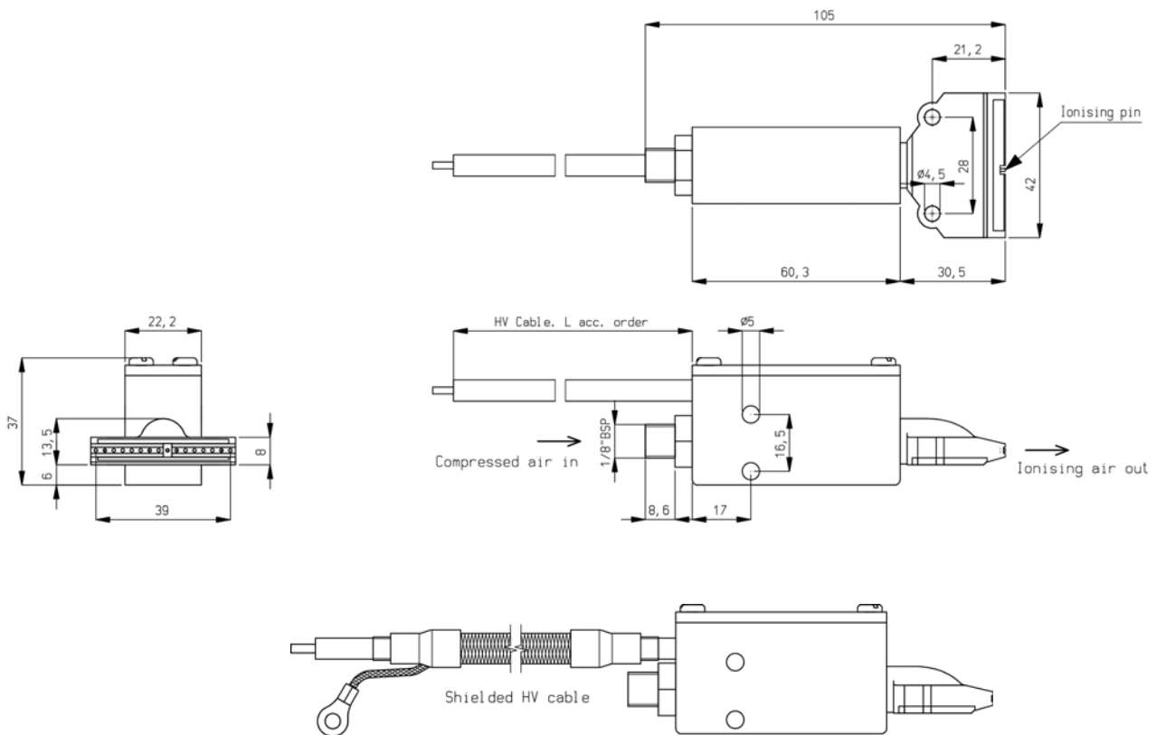
Afbeelding 1: ionisatiesproeier type FLAT 2
