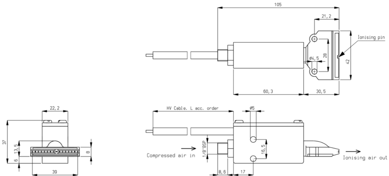
Abbildung 1: Ionensprühdüse Typ FLAT 2
