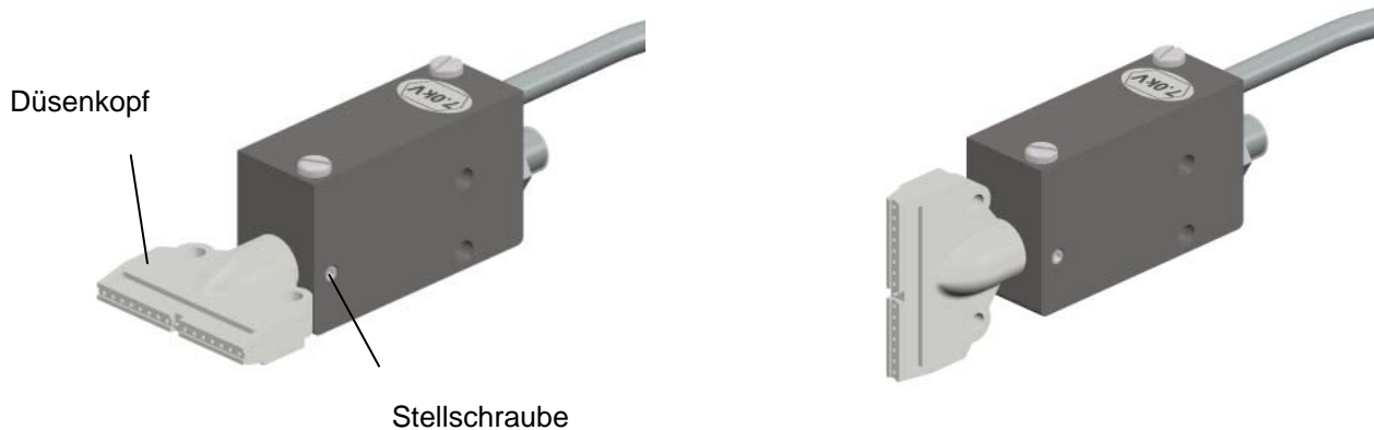
Abbildung 3: Drehen des Düsenkopfs
