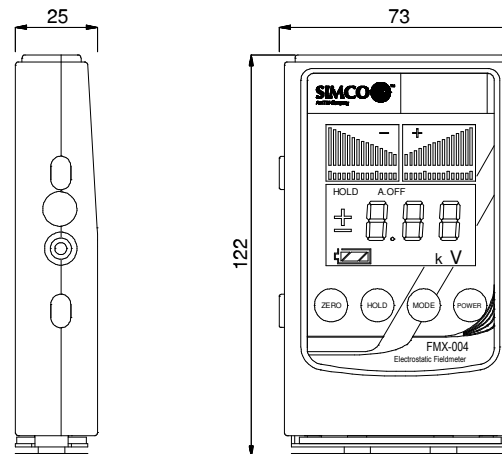
Zeichnung FMX-004
